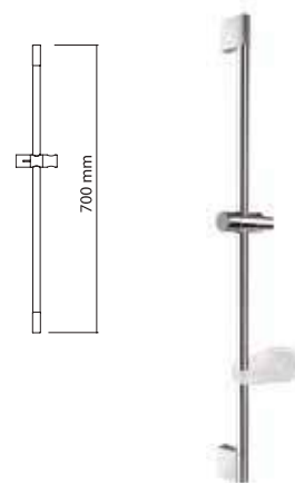
MALAWI ø20x700 mm BARRA DE DUCHA Sliding bar Barre de douche
