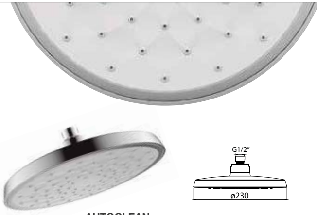
AUTOCLEAN Ø230 mm
