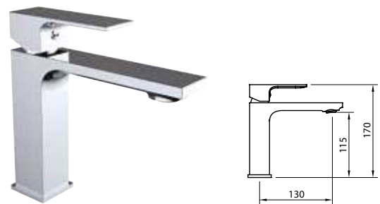
LAVABO 115 Basin mixer 115 | Mitigeur lavabo 115
