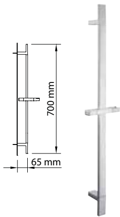
TREND 30x10x700 mm BARRA DE DUCHA Sliding bar Barre de douche
