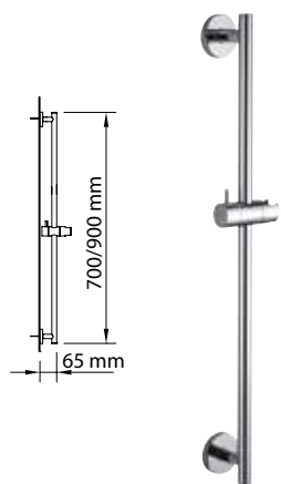
STYLE BARRA DE DUCHA Sliding bar Barre de douche
