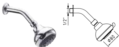
ZANZIBAR Ø80 mm
