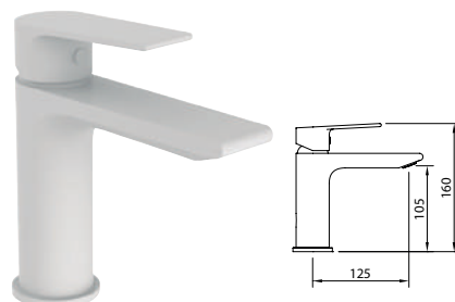
AGORA xtreme MITIGEUR LAVABO BLANC MAT 105 Matte white basin mixer 105
