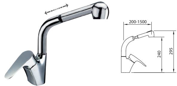
HABANA xtreme 240 mm MITIGEUR ÉVIER DOUCHETTE EXTRACTIBLE Pull-out sink mixer
