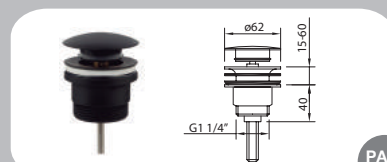
LEO NEGRO MATE _ 60702 Vidage Universel. Métallique Universal drain quick-clac. Metallic
