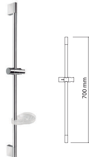
MALAWI ø20x700 mm BARRE DE DOUCHE Sliding bar
