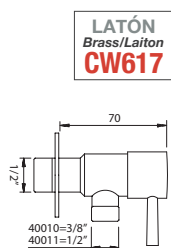
DESIGN ROBINET D'ÉQUERRE Angle valve
