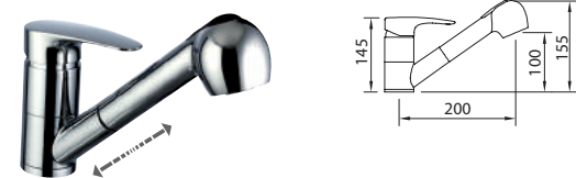
BAHAMA xtreme 100 mm MITIGEUR ÉVIER DOUCHETTE EXTRACTIBLE Pull-out sink mixer
