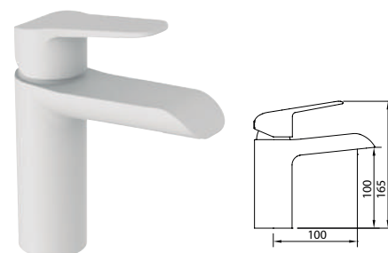
START elegance MITIGEUR LAVABO BLANC MAT 100 Matte white tall basin mixer 100
