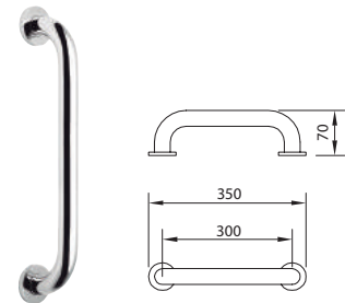
BARRE DE SÉCURITÉ Brass chrome security curve handle
