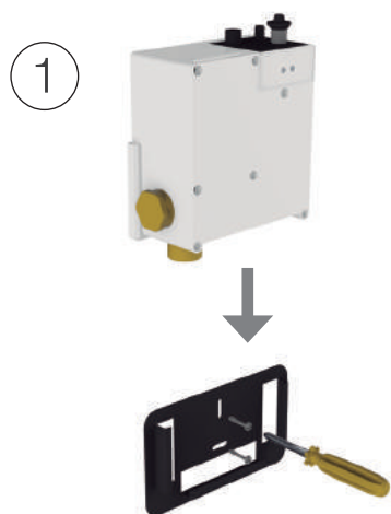
Fixation du boîtier Wall box fixing
