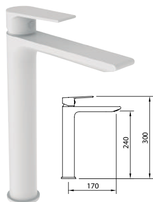
AGORA xtreme MITIGEUR LAVABO BLANC MAT 240 Matte white tall basin mixer 240
