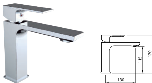
MITIGEUR LAVABO 115 Basin mixer 115
