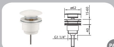
LEO BLANCO MATE _ 60701 Vidage Universel. Métallique Universal drain quick-clac. Metallic
