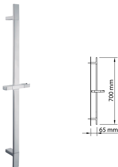
TREND 30x10x700 mm BARRE DE DOUCHE Sliding bar
