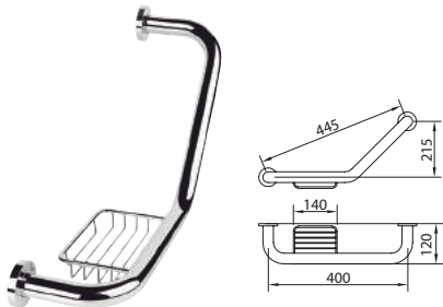
BARRE DE SÉCURITÉ AVEC PORTE-SAVON Brass chrome security curve handle with soap dish 40cm
