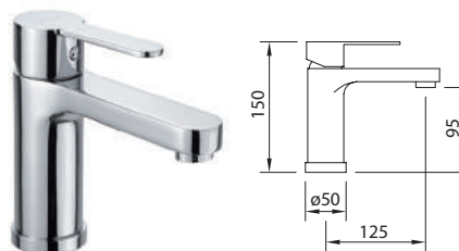
MITIGEUR LAVABO 95 Basin mixer 95
