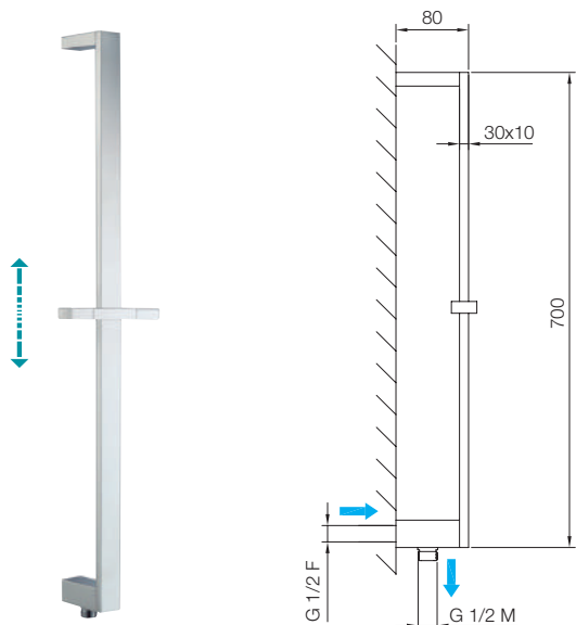
TREND - 30x10x700 mm BARRE DE DOUCHE ENCASTRÉ Concealed sliding bar
