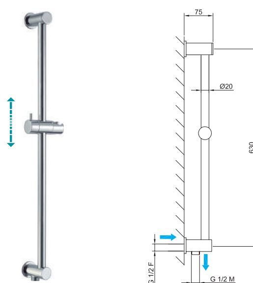
CITY - Ø20x715 mm BARRE DE DOUCHE ENCASTRÉ Concealed sliding bar
