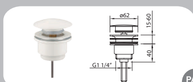
LEO BLANCO MATE _ 60701 Vidage Universel. Métallique Universal drain quick-clac. Metallic
