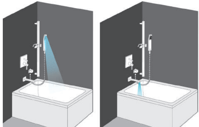
Bain-Douche encastrée avec inverseur. Pomme de douche ou douchette et bec. Concealed bath-shower with diverter. Handset and spout.
