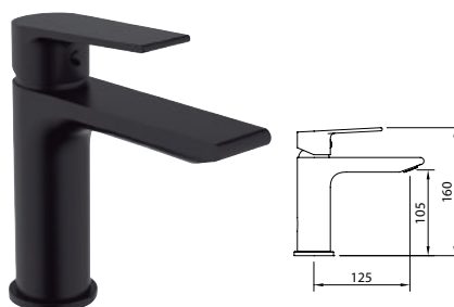
AGORA Xtreme MITIGEUR LAVABO NOIR MAT 105 Matte black basin mixer 105
