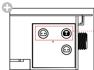
Connexion du capteur Sensor tap connection
