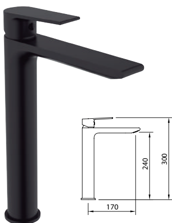
AGORA Xtreme MITIGEUR LAVABO NOIR MAT 240 Matte black tall basin mixer 240
